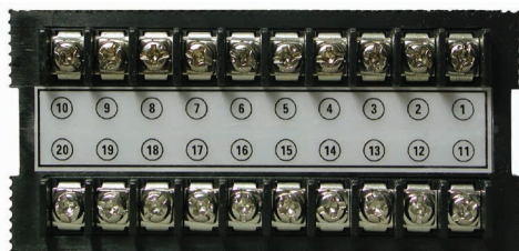
Рис. 7 – Вид прибора сзади
