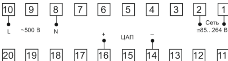
Рис. 4 – Клеммы подключения P94-V-1-0.5-1420
