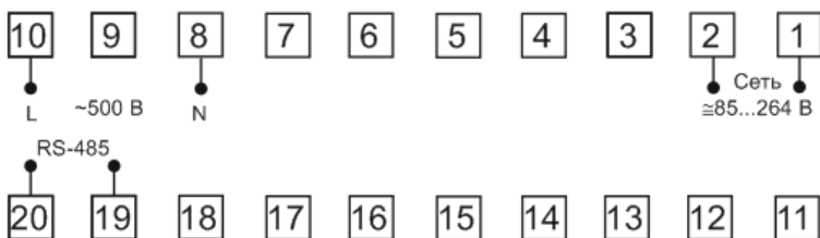
Рис. 5 – Клеммы подключения P94-V-1-0.5-RS485
