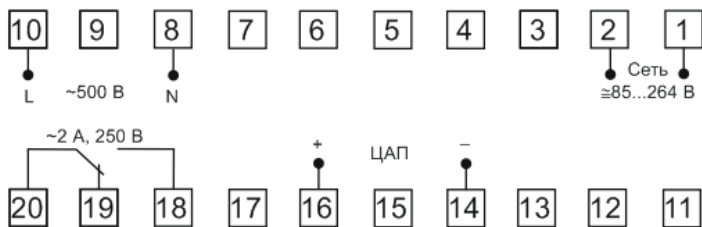
Рис. 6 – Клеммы подключения P94-V-1-0.5-K-1420
